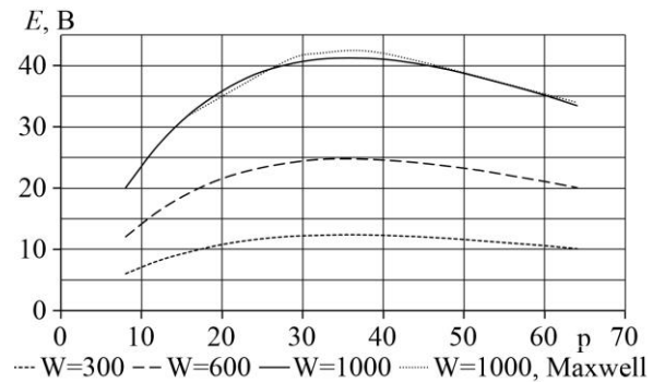
Рис. 14. Зависимость ЭДС от числа полюсов статора. 14
