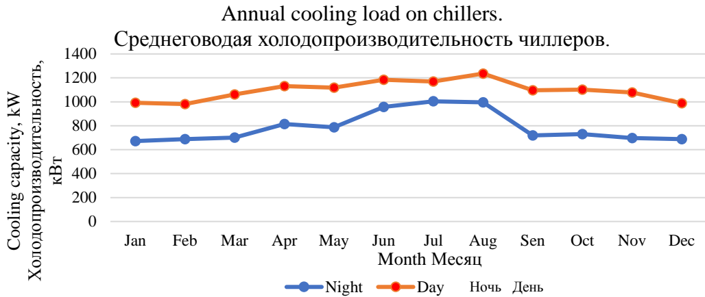
Рис.4. Дневная и ночная среднегодовые нагрузки. 6
