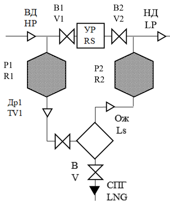
Рис.5. Схема получения СПГ с очисткой сырьевого газа в регенеративных теплообменниках. 7
