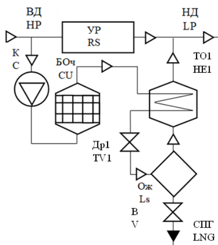
Рис.2. Технологическая схема получения СПГ в простом дроссельном цикле высокого давления. 4
