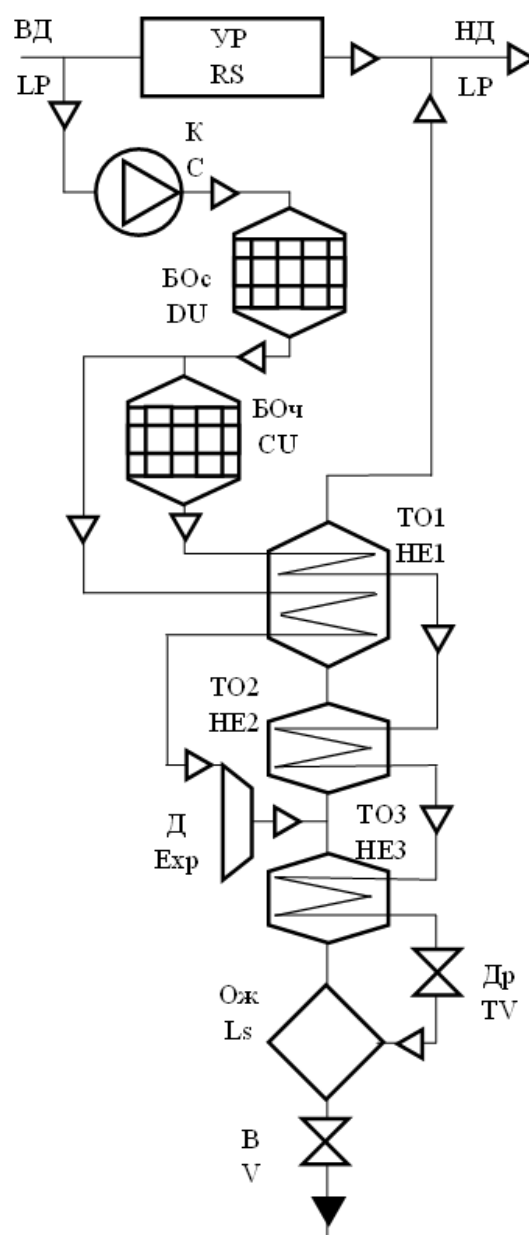
Рис.3. Схема производства СПГ на ГРС по циклу среднего давления [7]. 5
