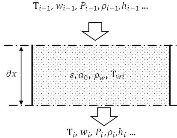
Рис. 6. Физическая модель регенеративного теплообменного аппарата. 8
