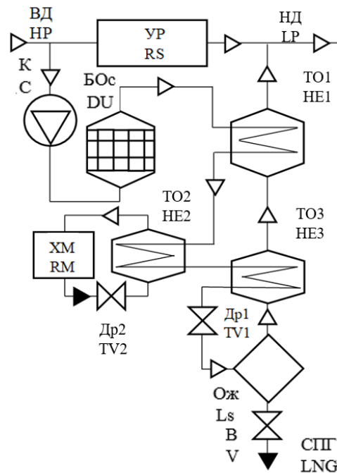
Рис.4. Общая технологическая схема высокого давления с холодильной машиной. 6
