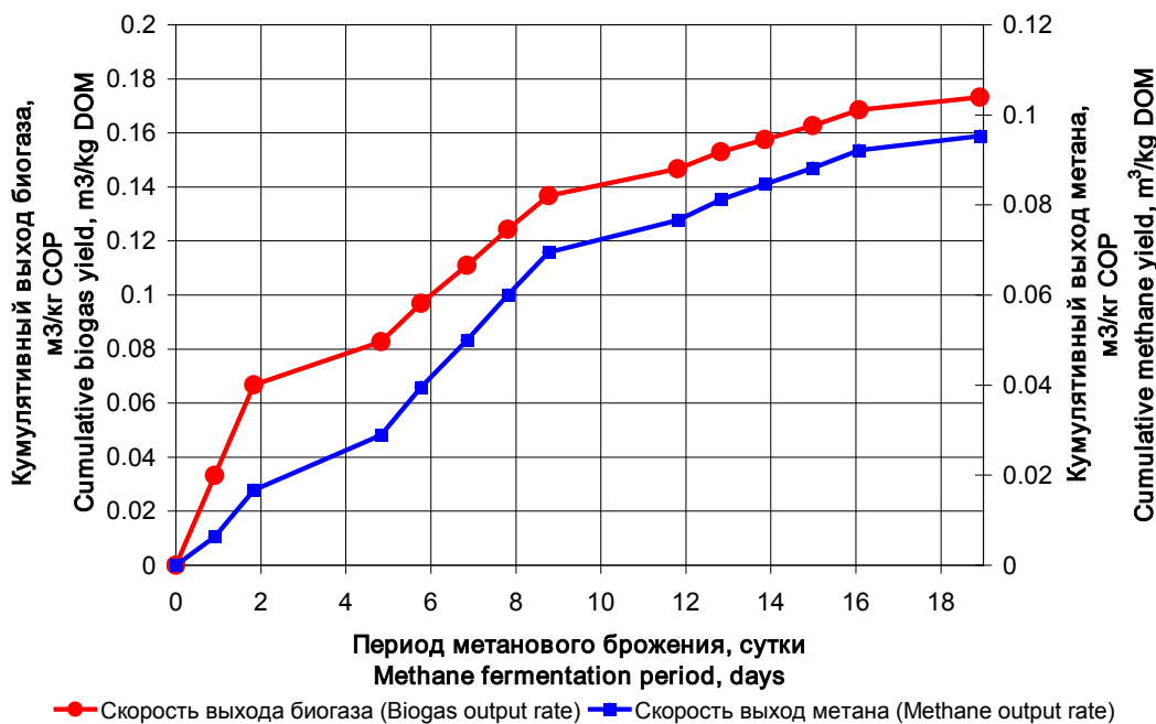
Рис. 7. Кумулятивный выход биогаза и метана при метановом сбраживании смеси навоза крупного рогатого скота с яблочными выжимками (30.7% по СОВ) в мезофильном режиме при температуре 36±1°С. 9
