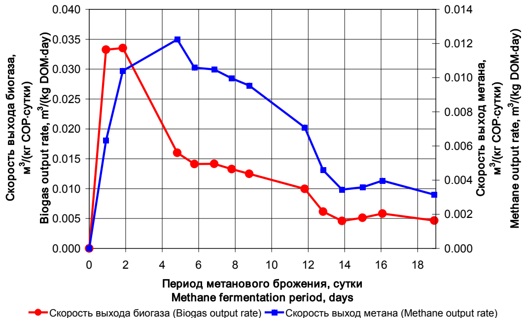
Рис. 6. Динамика изменения скорости выхода биогаза при метановом сбраживании смеси навоза крупного рогатого скота с яблочными выжимками (30.7% по СОВ) в мезофильном режиме при температуре 36±1°С. 8
