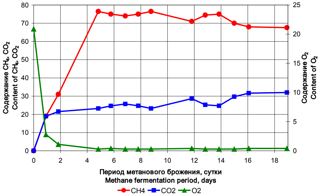
Рис. 9. Изменение состава биогаза во времени при сбраживании смеси навоза крупного рогатого скота с яблочными выжимками (30.7% по СОВ) в мезофильном режиме при температуре 36\pm 1^\circ\text{C} . 11
