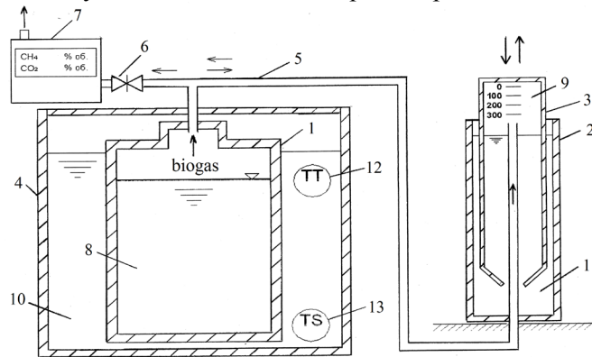
1 – емкость ферментера; 2 – неподвижная часть газгольдера; 3 – подвижная часть газгольдера; 4 – емкость с теплоносителем; 5 – трубка ПВХ; 6 – газовый кран; 7 – газоанализатор; 8 – рабочая среда ферментера; 9 – внутреннее пространство газгольдера с биогазом; 10 – теплоноситель (вода); 11 – 5% водный раствор NaCl; 12 – ртутный термометр; 13 – терморегулятор ( \Delta T = \pm 1^\circ C ).
