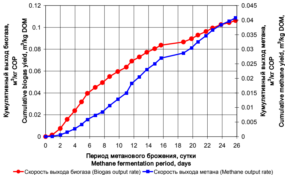
Рис. 2. Динамика изменения скорости выхода биогаза и метана при метановом сбраживании смеси навоза крупного рогатого скота с яблочными выжимками (28.1% по СОВ) в психрофильном режиме при температуре 22\pm 1^\circ\text{C} . 3
