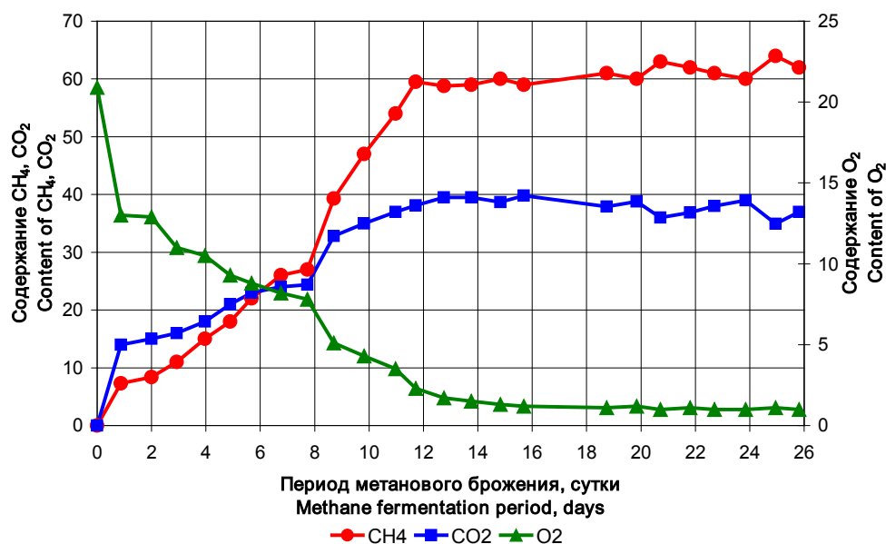
Рис. 5. Изменение состава биогаза во времени при сбраживании смеси навоза крупного рогатого скота с яблочными выжимками (28.1% по СОВ) в психрофильном режиме при температуре 22±1°С. 6
